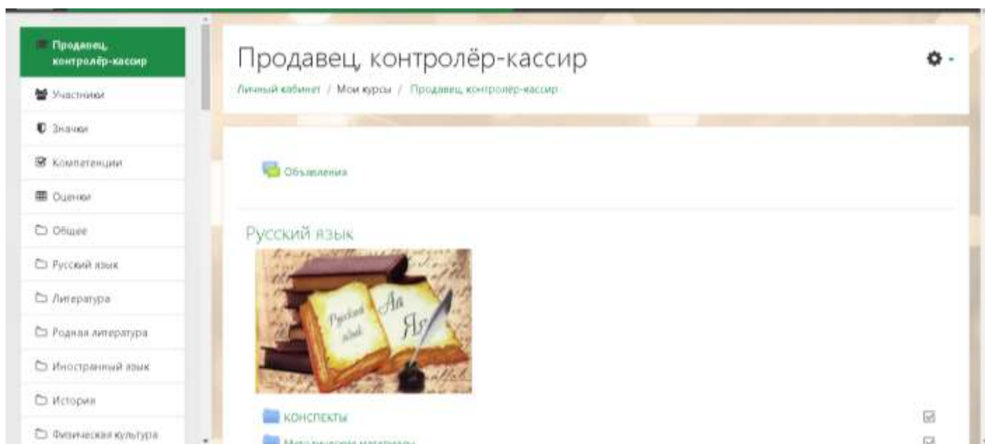
Рис. 4. Страница курса.
