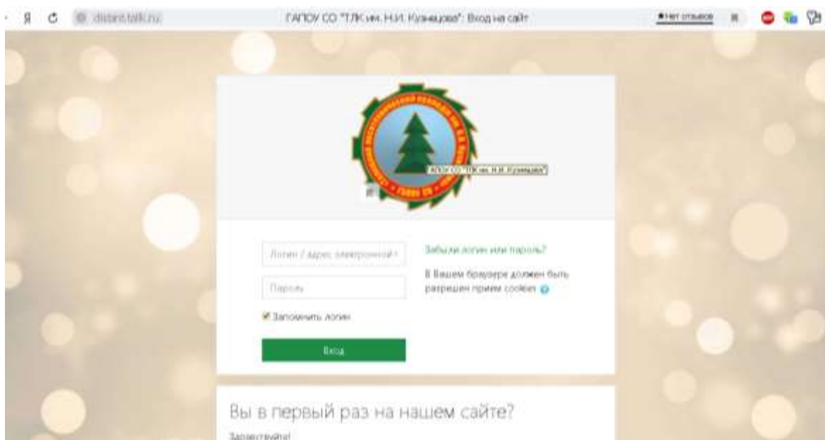
Рис. 2. Страница авторизации.
