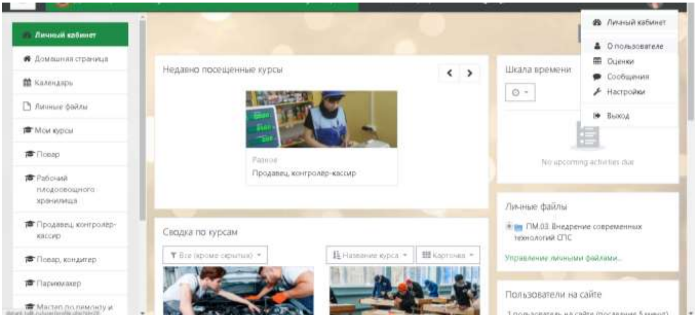
Рис. 5. Личный кабинет.
